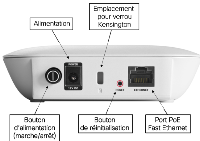
Figure 3. Panneau arrière du point d'accès Cisco WAP121 Wireless-N avec configuration par point unique
